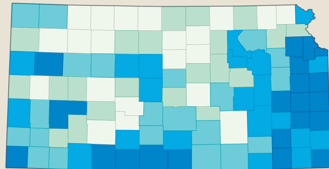
Quantile
